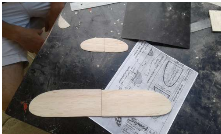
Figura 7 – Efetuando a Montagem do Protótipo
